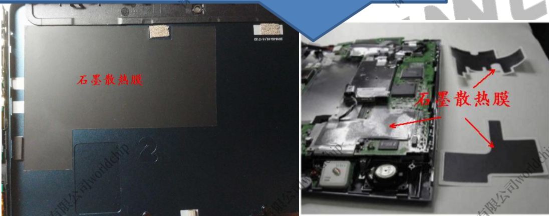
图 3-14 石墨散热膜实列示意
