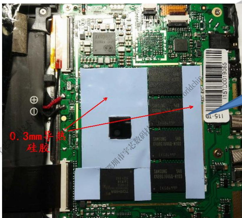
图 3-16 改善方案 (步骤 01)
