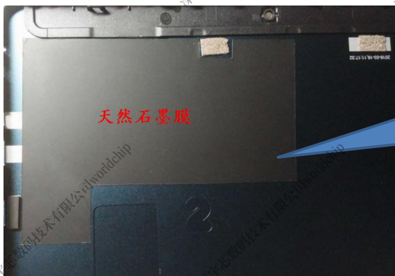
图 3-22 改善方案（步骤 07）
