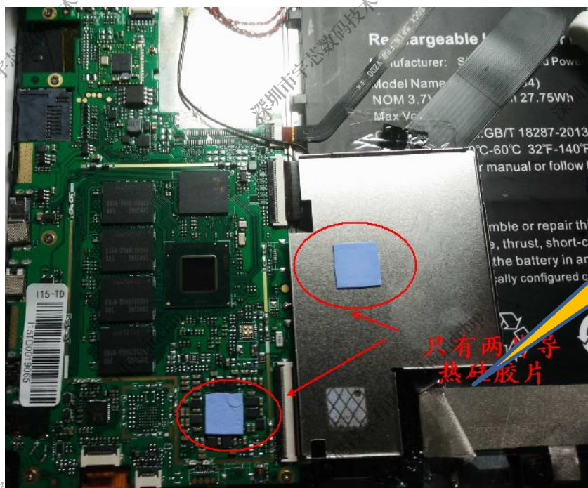
图 3-15 原始方案 (只贴硅胶)
