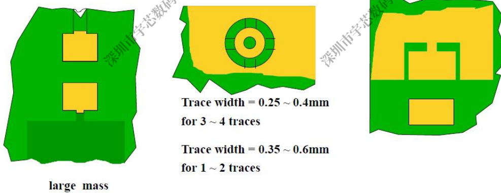
图 3-10 元器件地焊盘处理示意图
